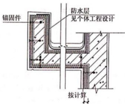
图 5.3.8 檐沟部位构造示意
