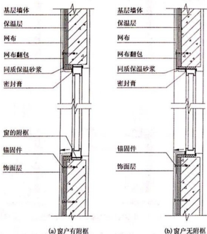
图 5.3.7-2 现浇系统非幕墙建筑门窗细部构造
