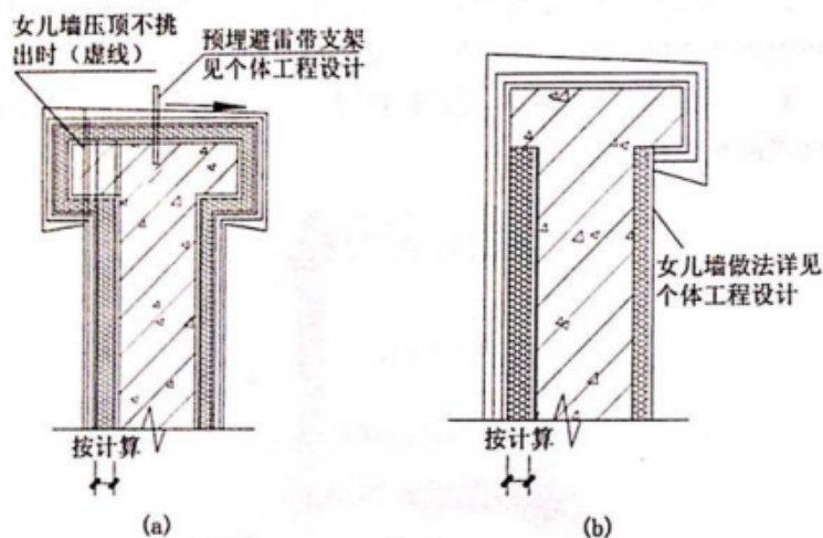
图 5.3.6 女儿墙部位构造示意
