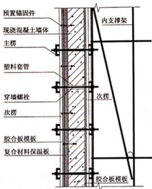
图 6.5.8 现浇系统支模方法示意
