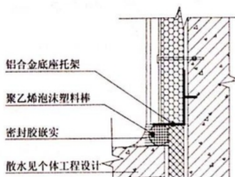
图 5.3.5 勒脚部位构造示意
