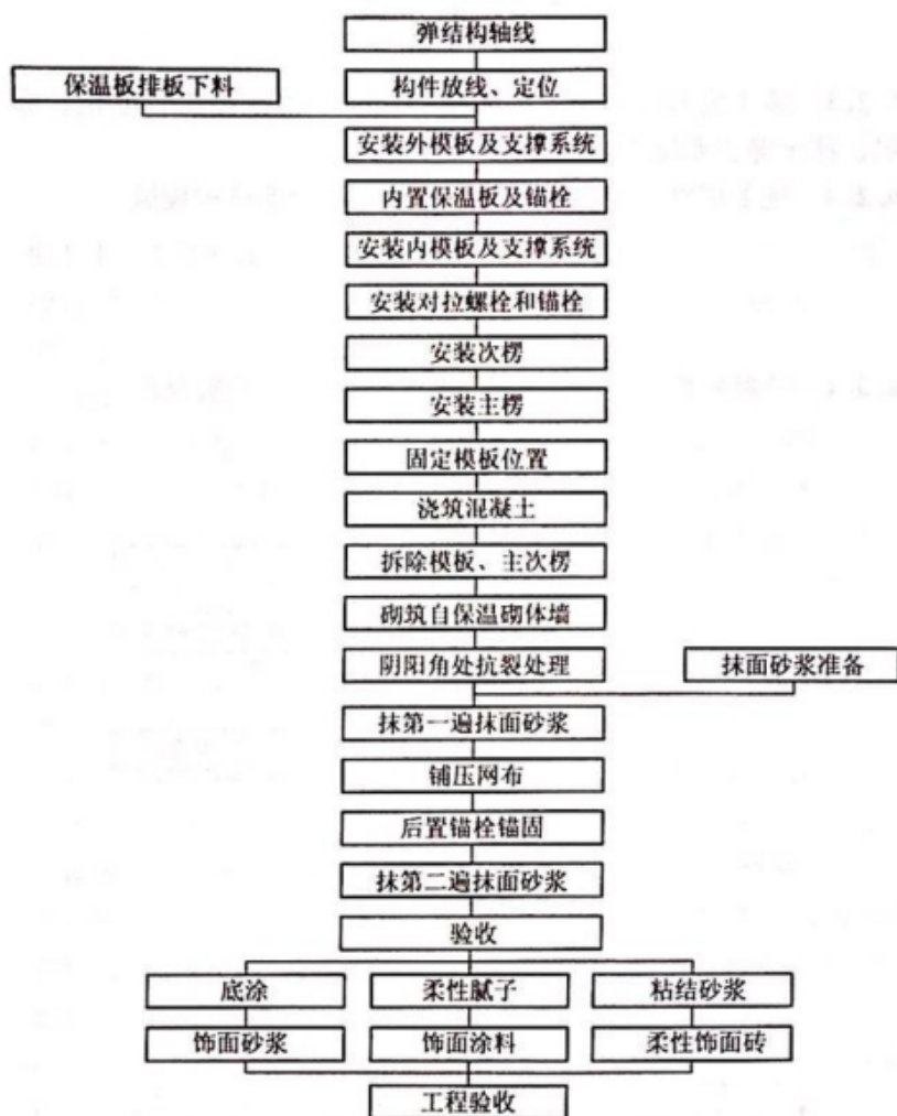
图 6.3.2 复合材料保温板现浇外墙外保温系统施工工艺流程
