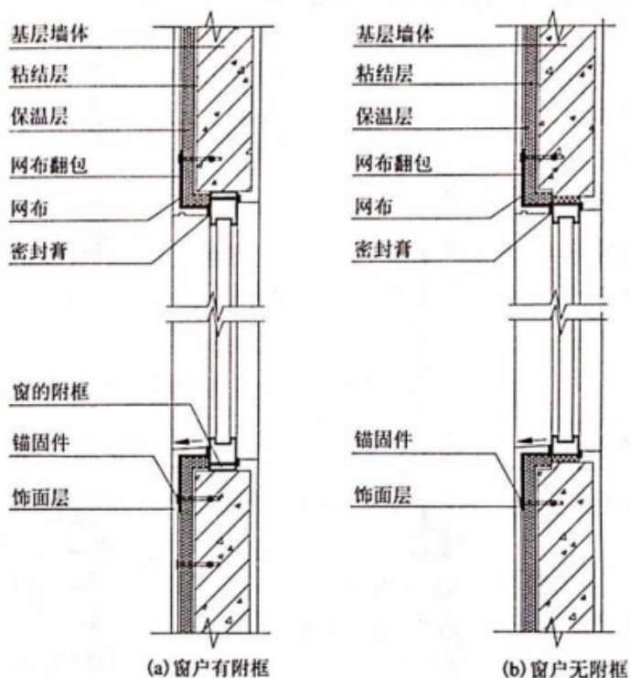
图 5.3.7-1 外贴系统非幕墙建筑门窗细部构造
