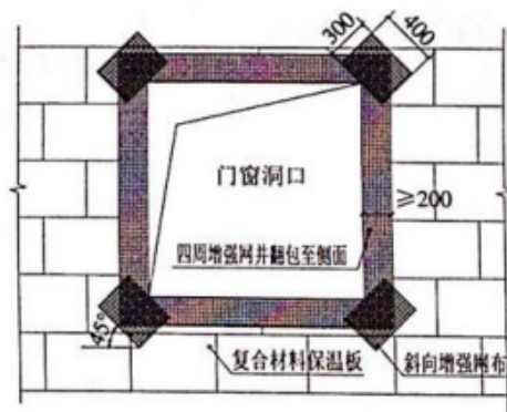
图 5.3.4 门窗洞口部位构造示意
