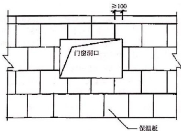
图 6.4.3-2 门窗洞口排板示意
