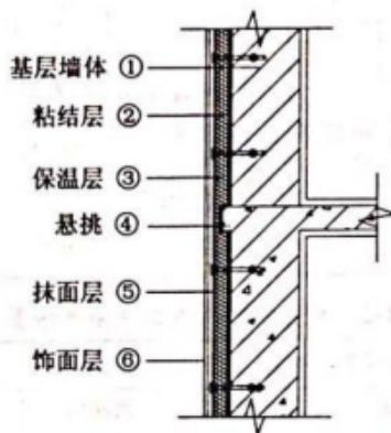
图 5.2.2 设置悬挑构造做法
